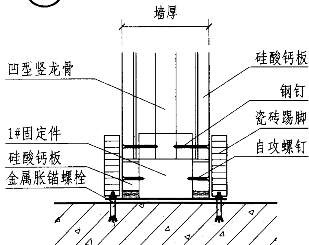
32 水泥踢脚或瓷砖踢脚
