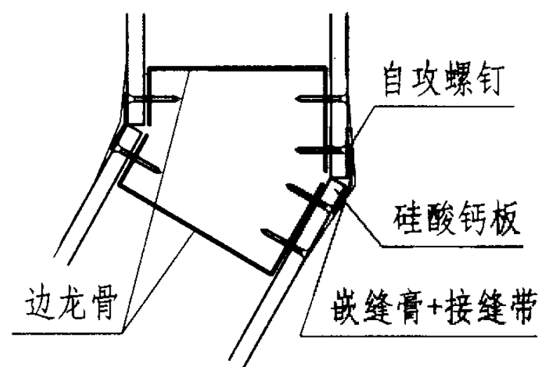
7 角板对接示意
