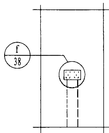
暗线插座立面
