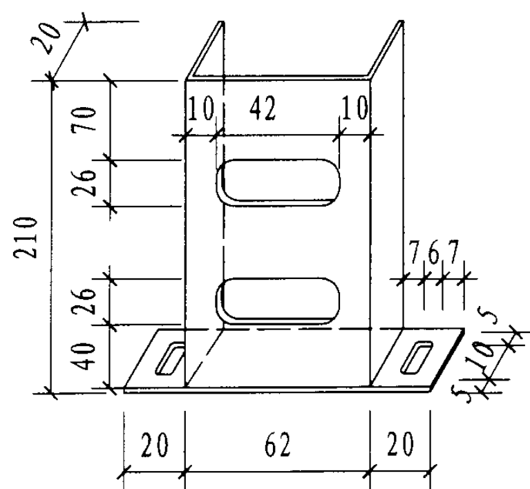
2#固定件
