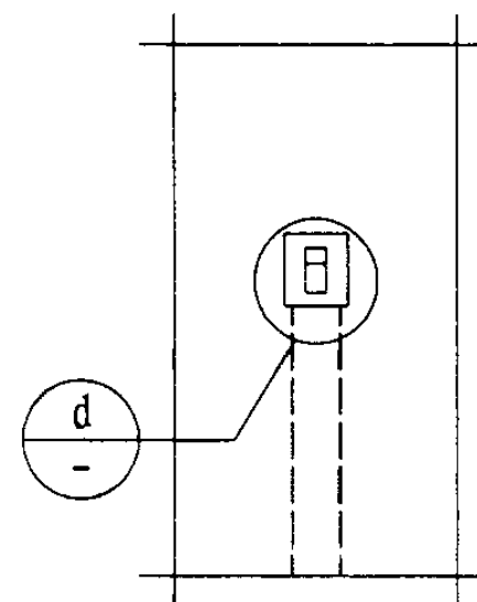
暗线开关立面
