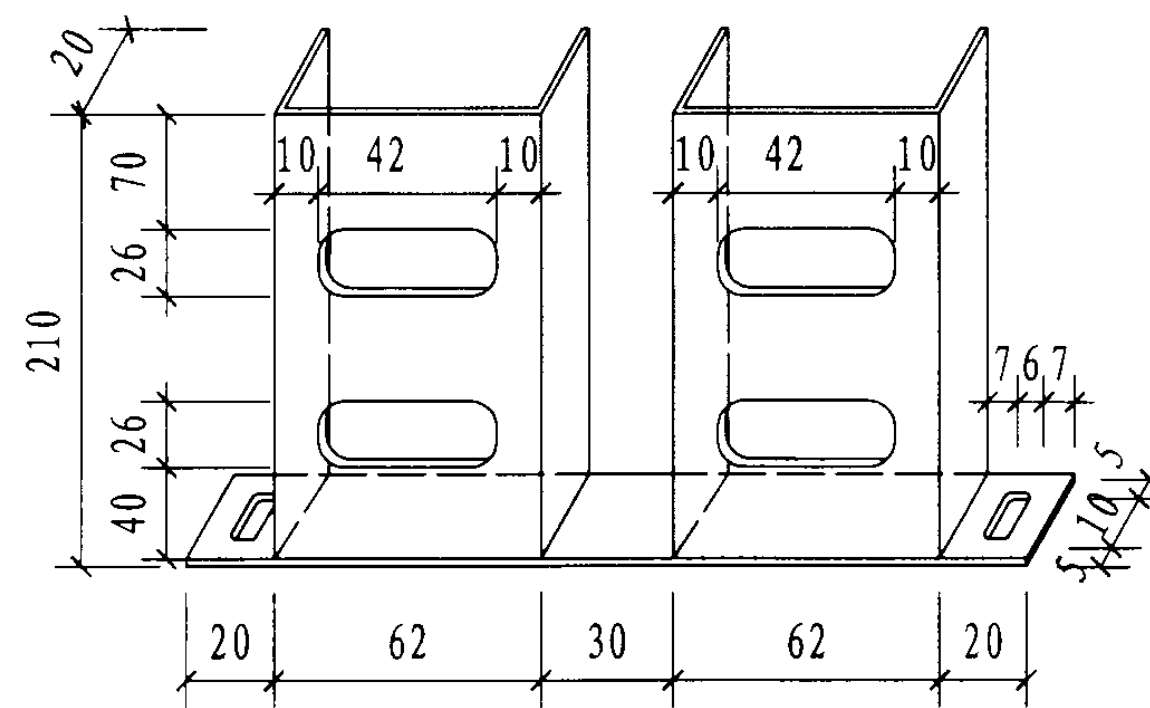
4#固定件
