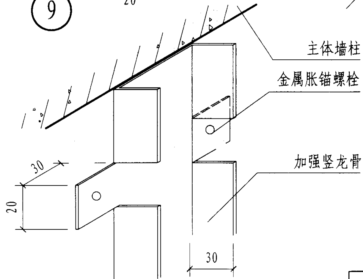
加强竖龙骨安装示意图
