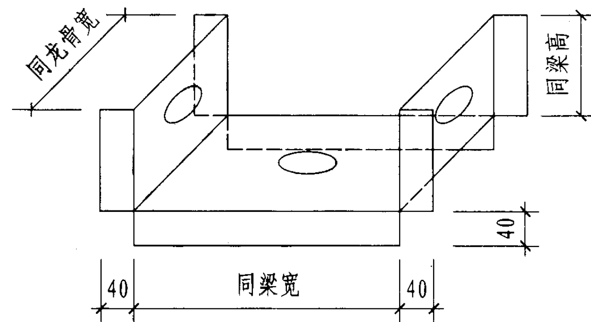
a 过梁卡 (镀锌钢板0.8厚)
