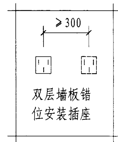
双层墙板插座立面
