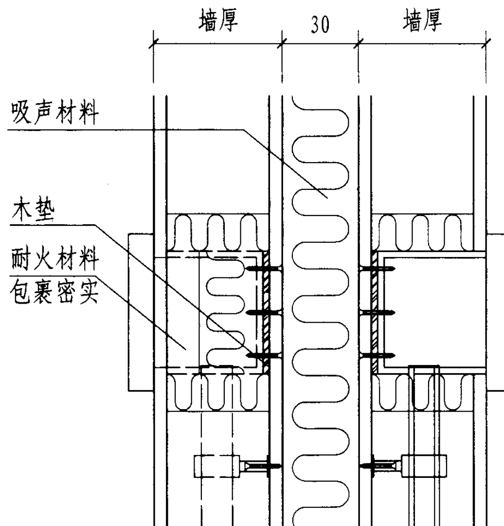
59 螺钉穿透管道托件示意
