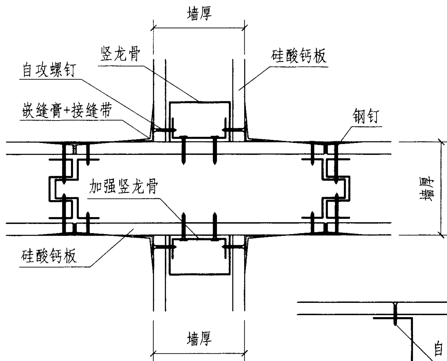
38 十字墙板连接
