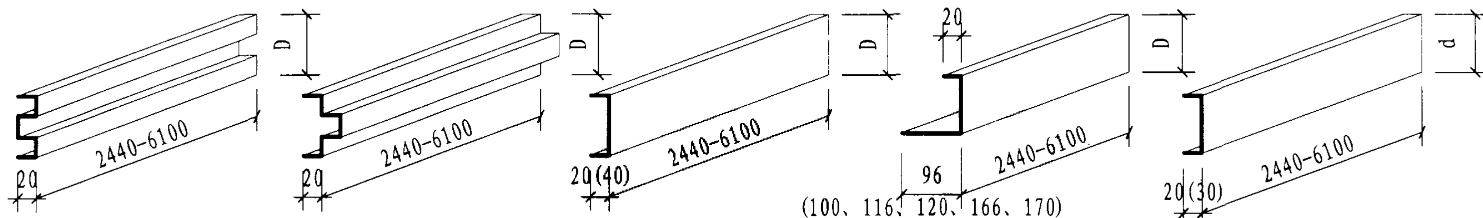
凹形竖龙骨
