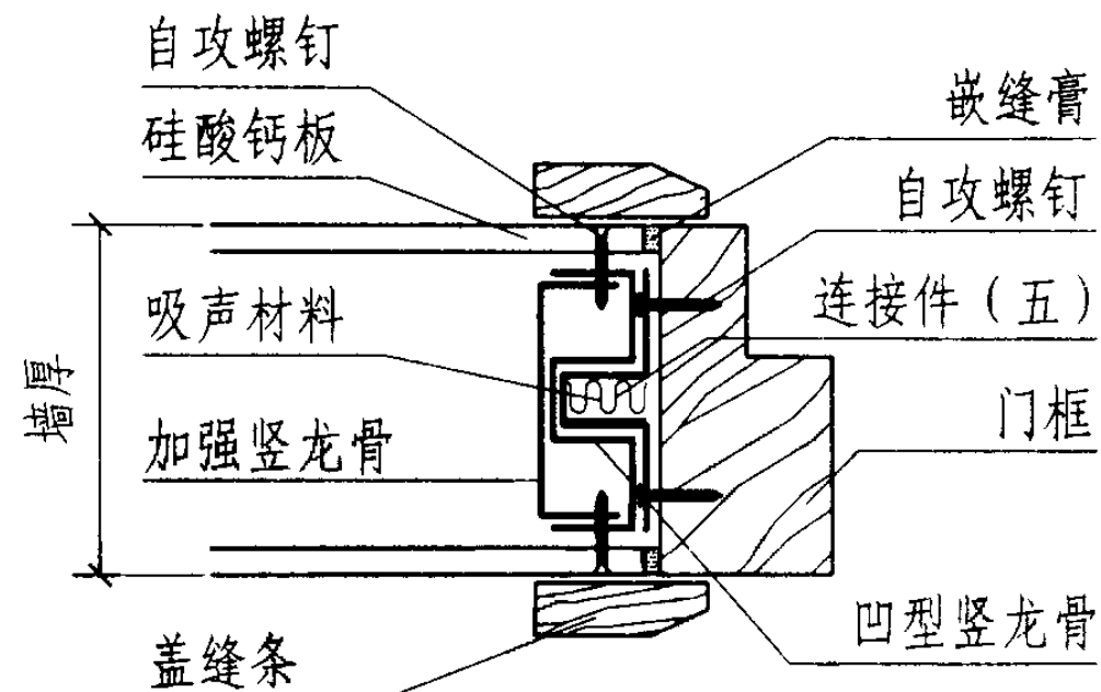
52 门框宽度 > 1000做法
