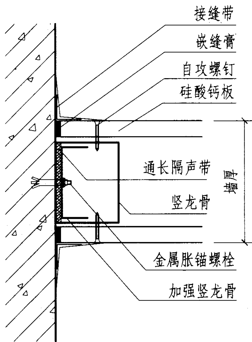
10 首板与主体墙柱连接
