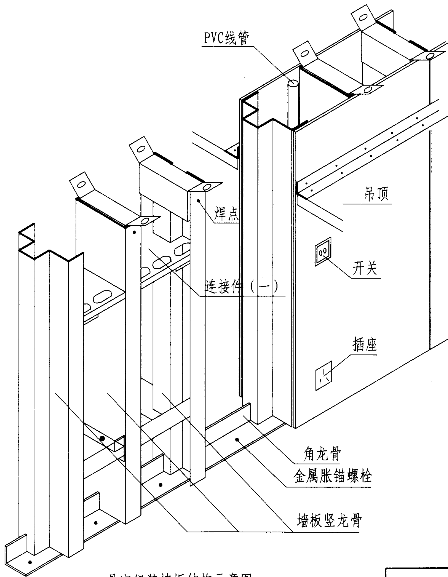
悬空组装墙板结构示意图
