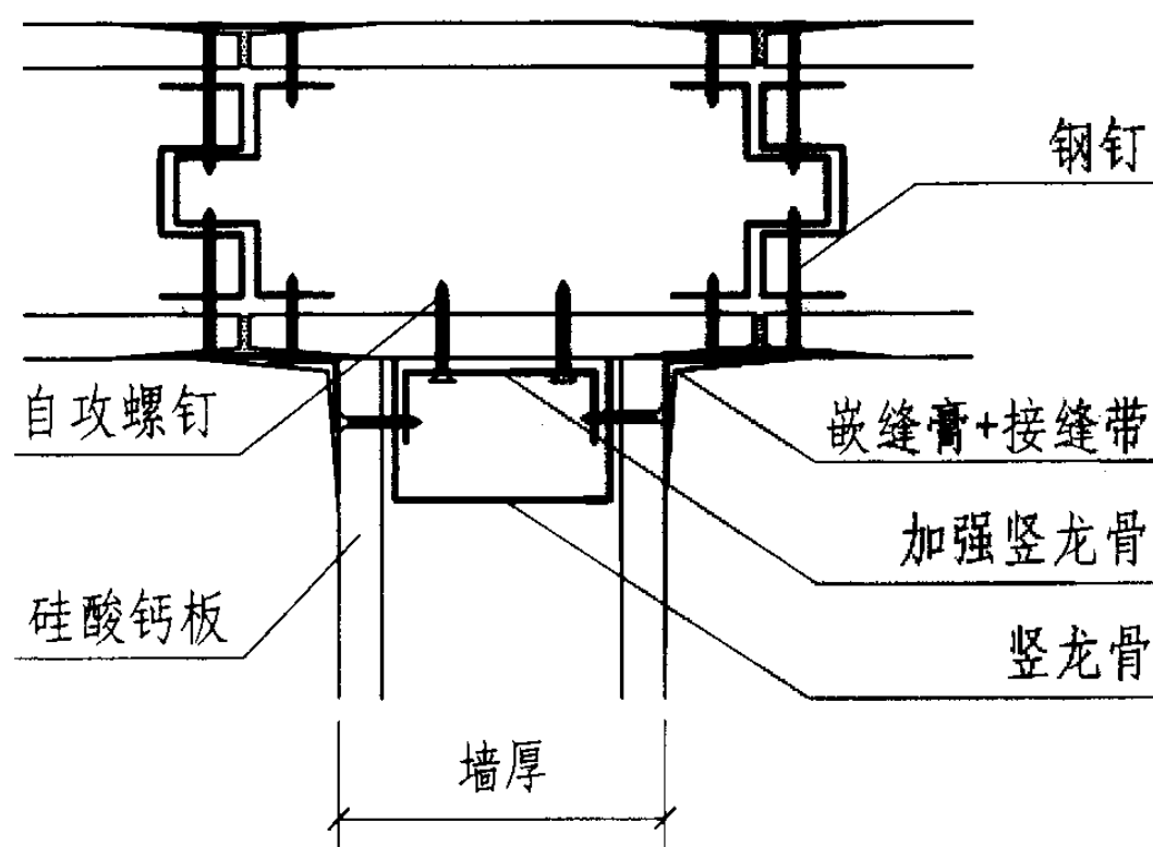
36 T形墙板连接
