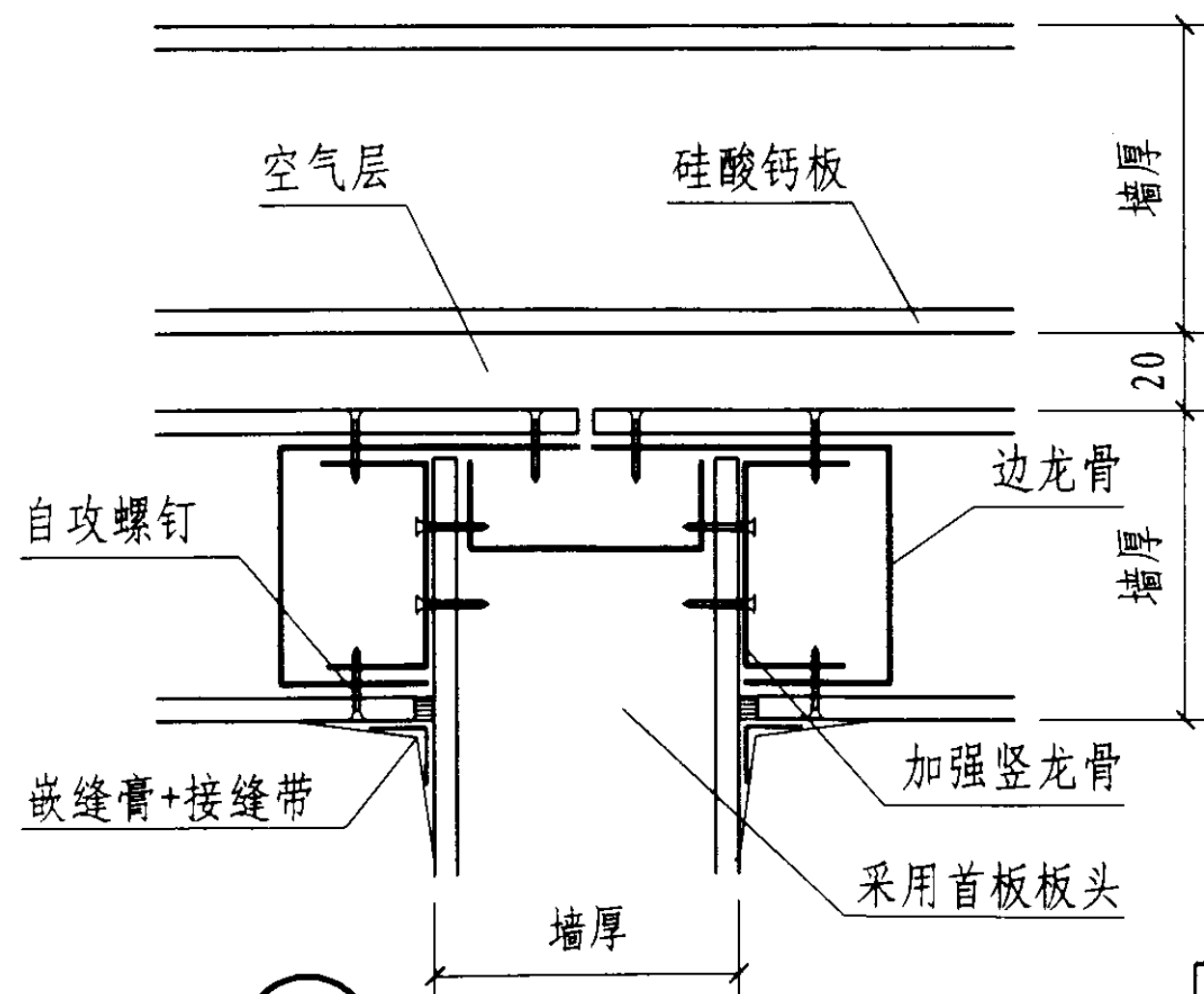
45 双层墙与单层墙连接
