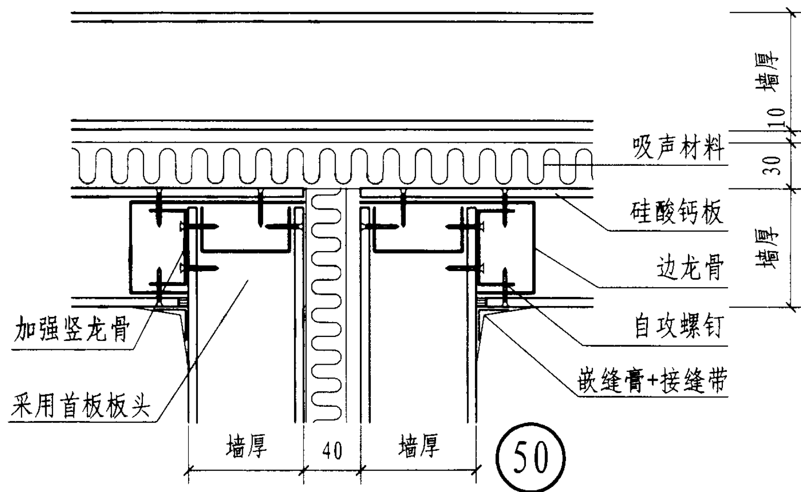
双层墙板连接节点 (二)
