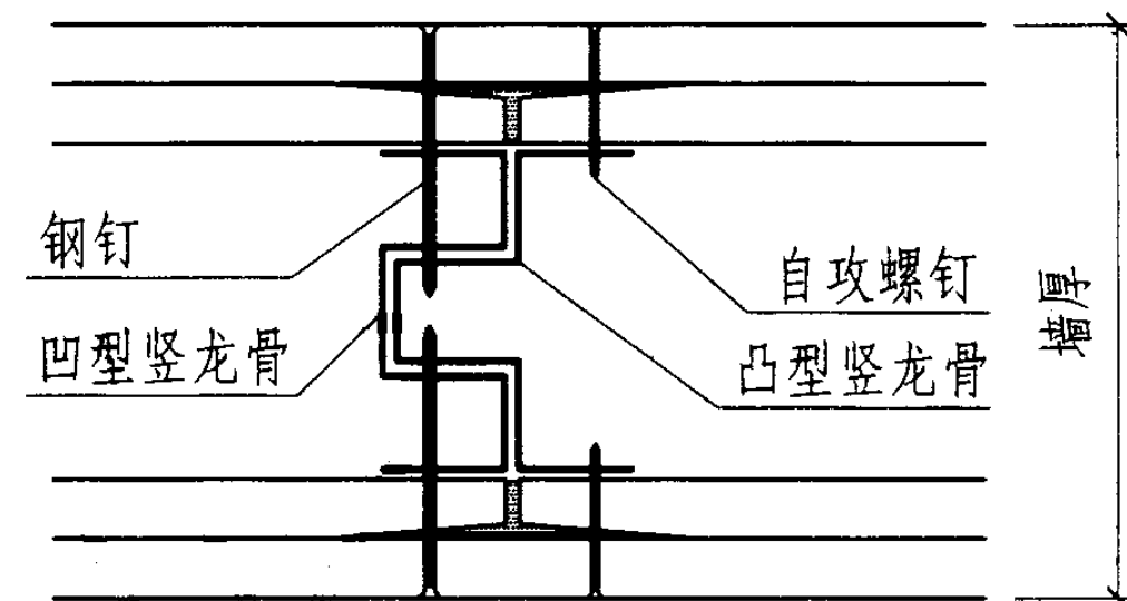
35 双层硅酸钙板接缝
