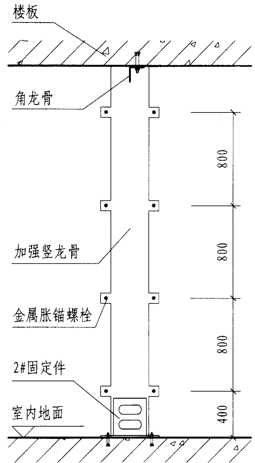
b 加强竖龙骨立面图
