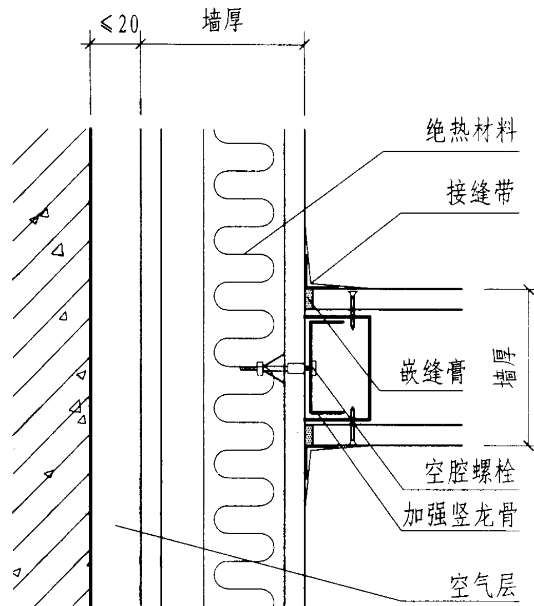
12 墙板与保温墙连接
