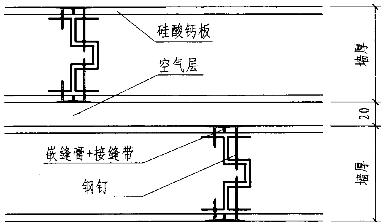
44 双层墙一字连接
