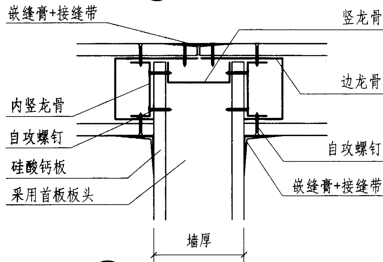
37 T形墙板连接
