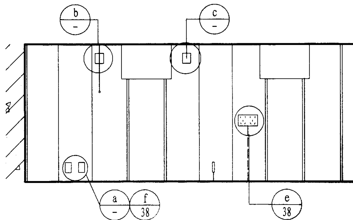
电气开关插座立面
