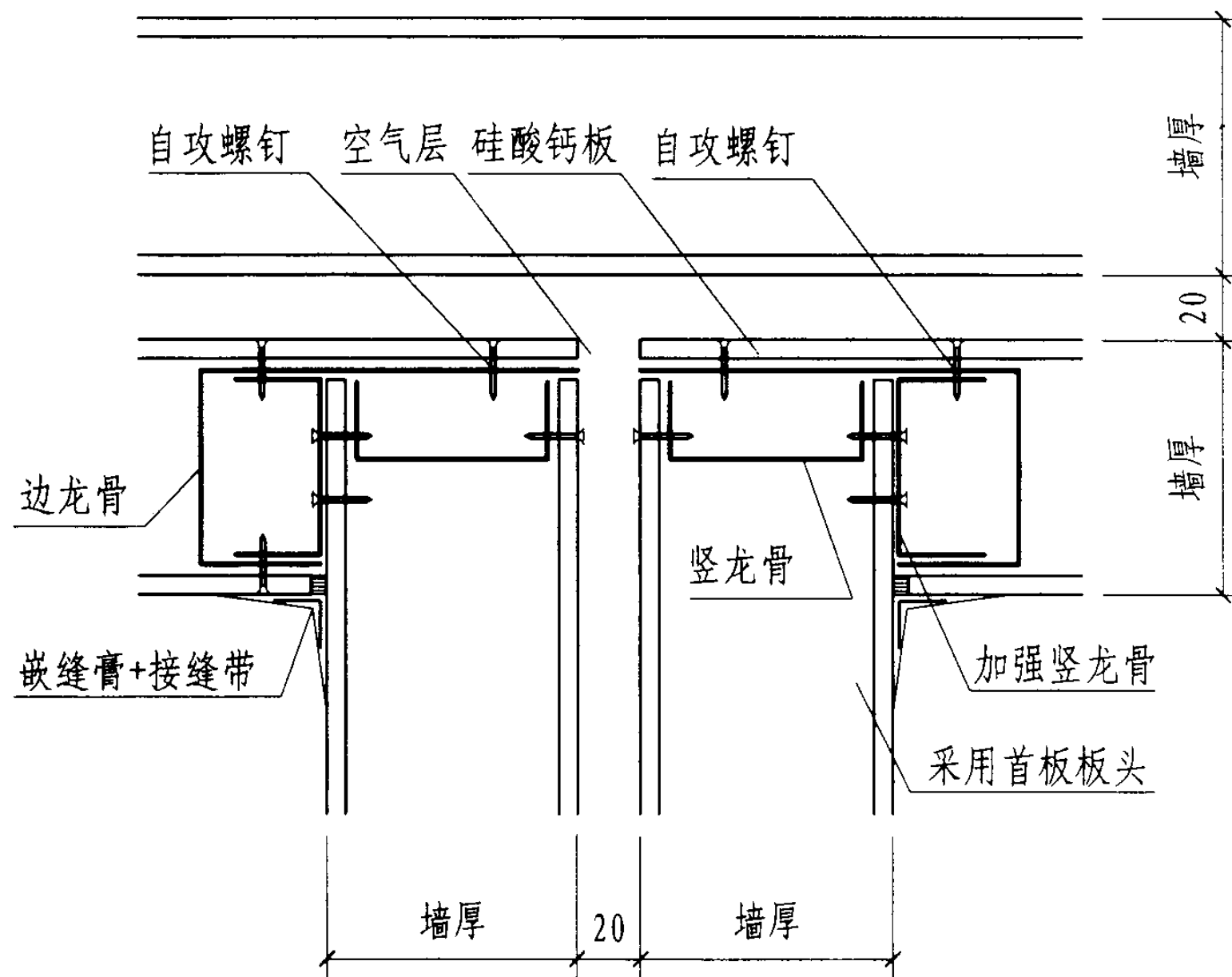
46 双层墙连接
