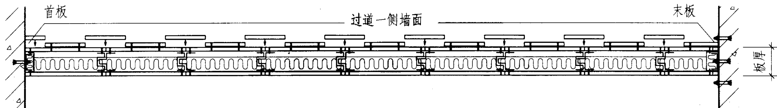
5 过道板组装示意图
