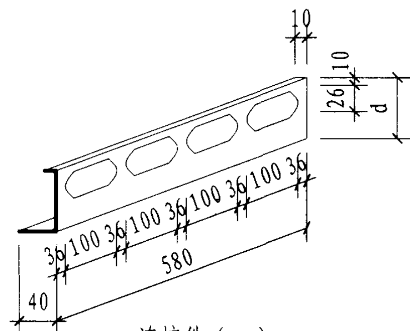
连接件 (一)
