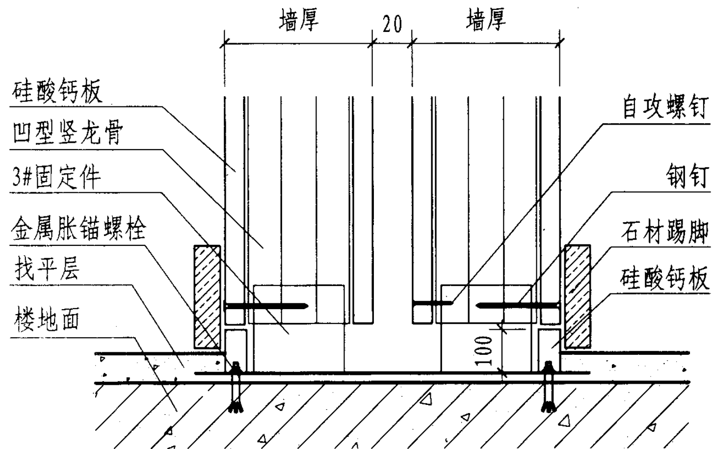
31 石材踢脚
