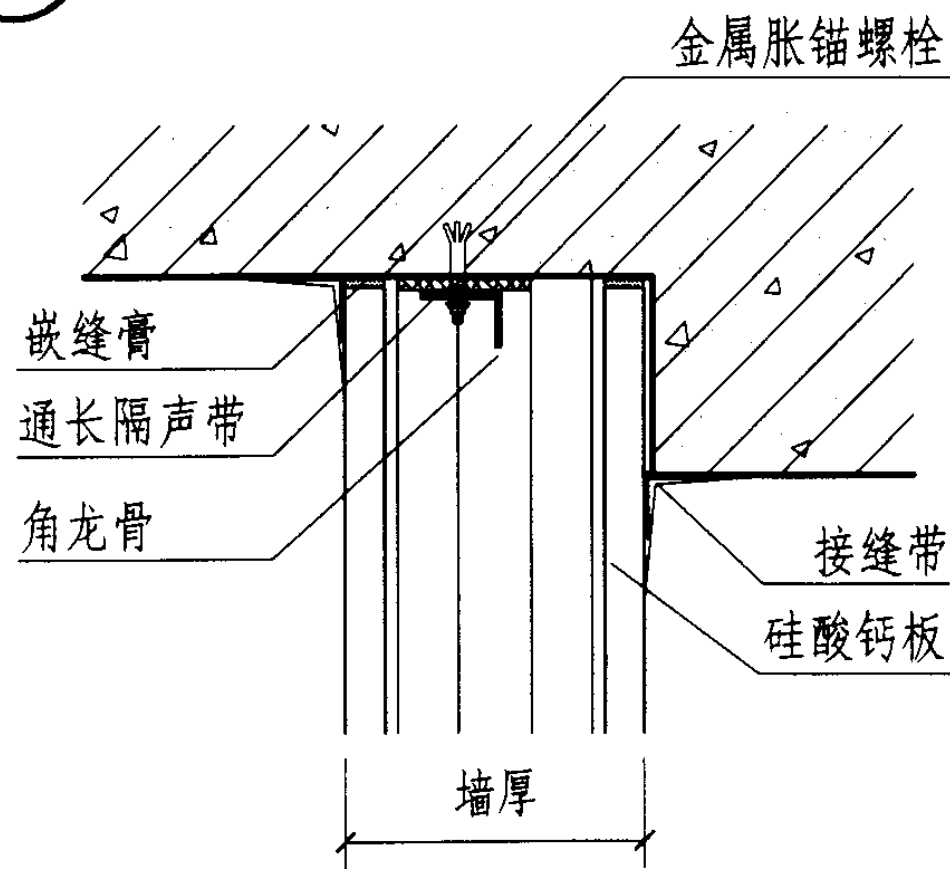
22 墙板沿梁与楼板顶面连接
