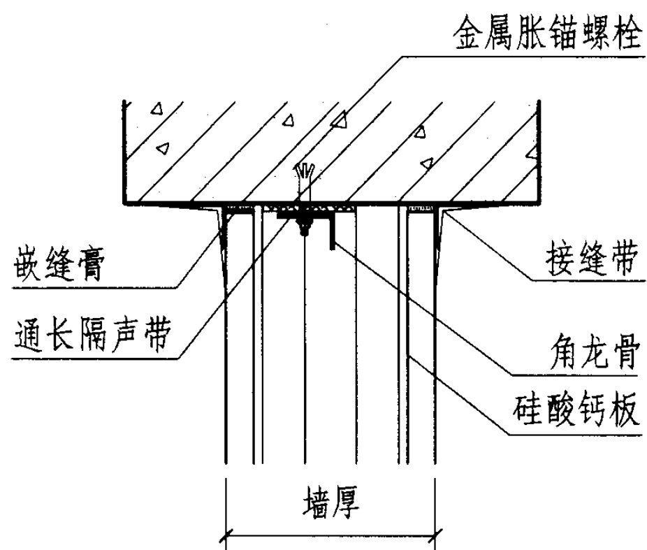
20 墙板与梁底连接
