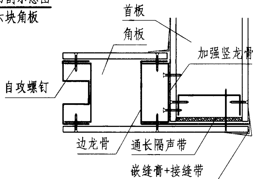
8 角板与首板连接
