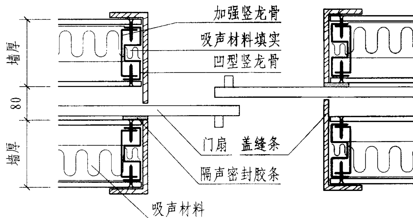
54 墙板与推拉门做法
