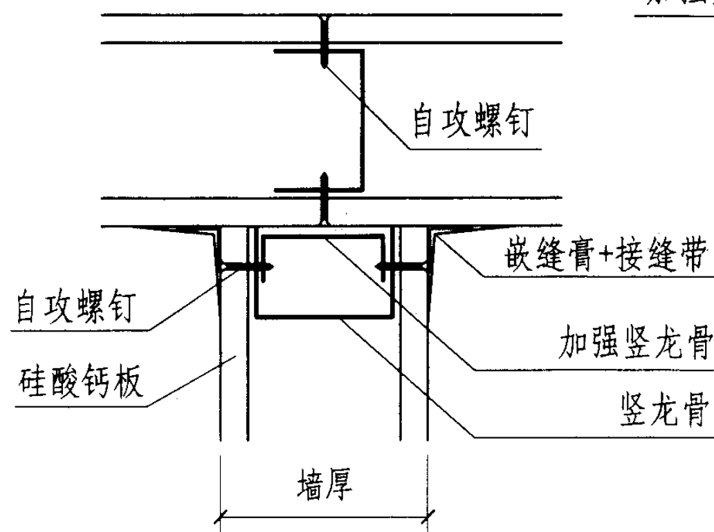
40 T形墙板连接
