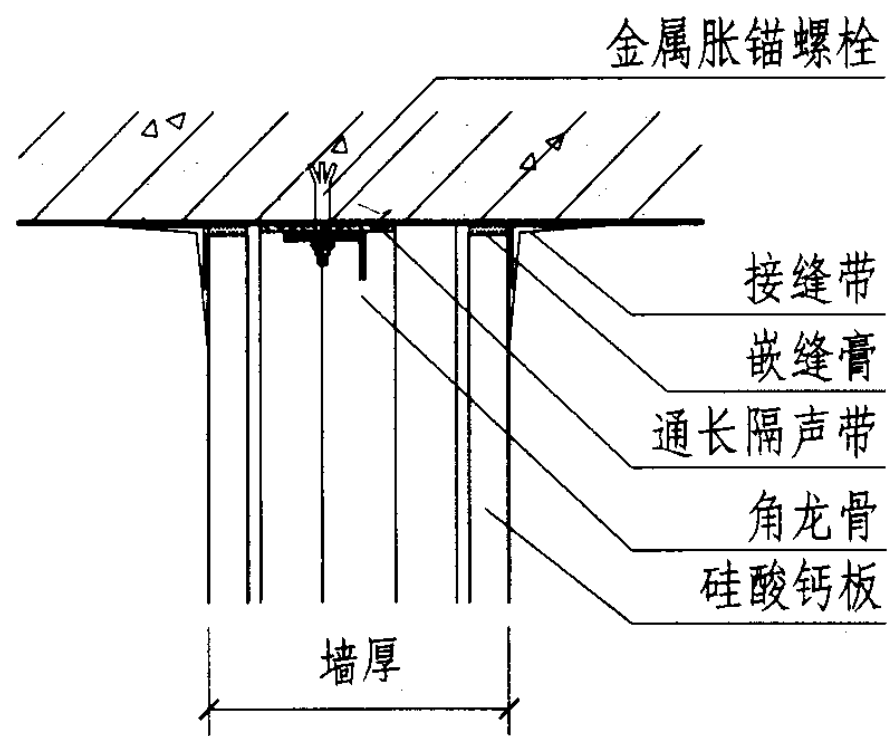
19 墙板与楼板顶面连接
