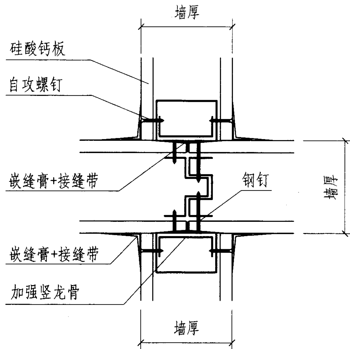
39 十字墙板连接
