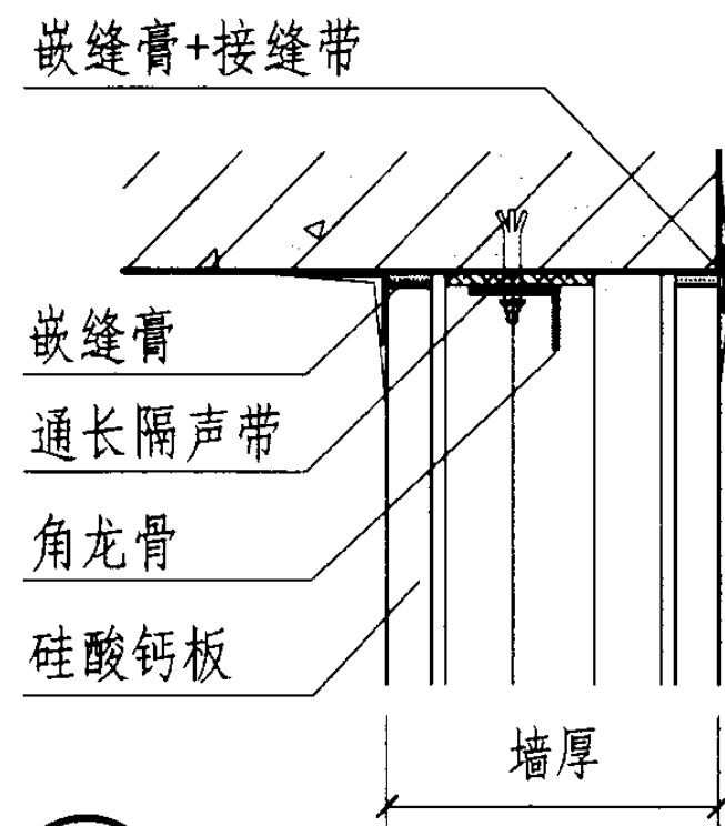
21 墙板与梁底一侧平齐连接
