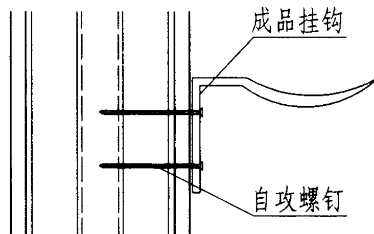
59 螺钉穿透管道托件示意
