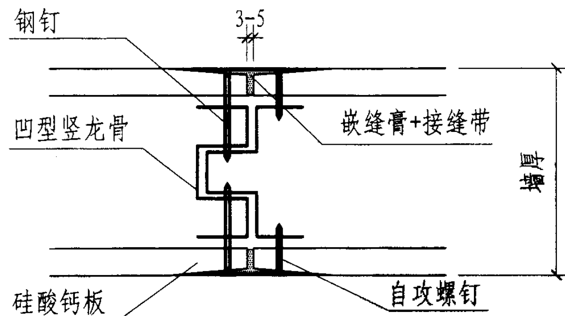
34 一字形墙板连接
