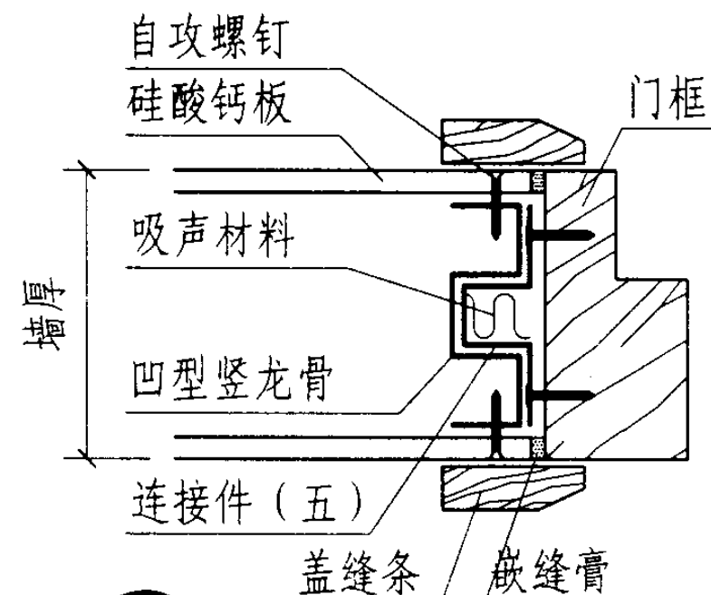
53 门框宽度 < 1000做法
