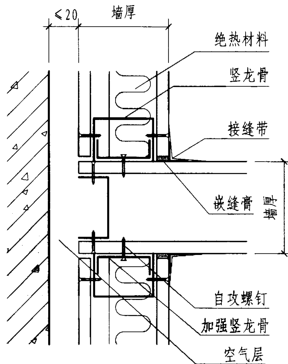
11 墙板与保温墙连接
