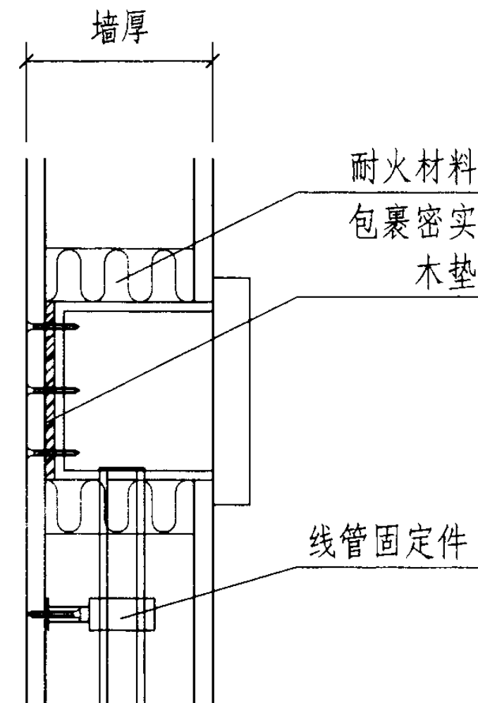
e 暗线插座
