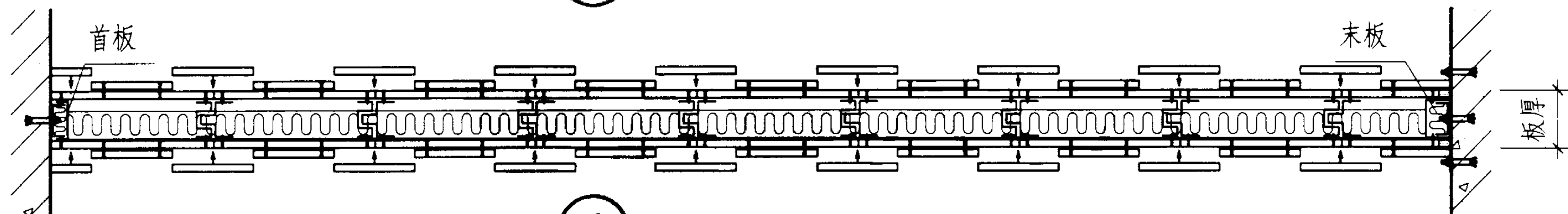
5 过道板组装示意图
