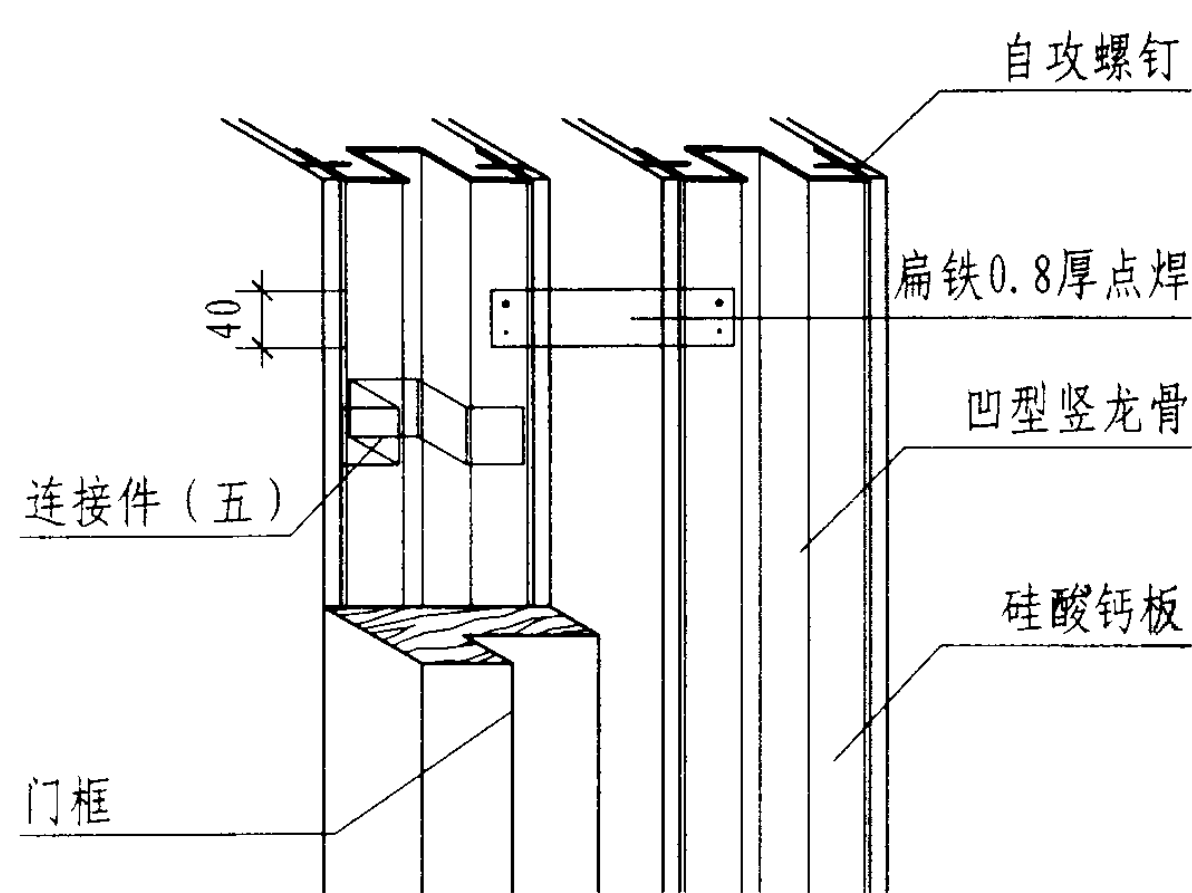
墙板与门框连接示意图
