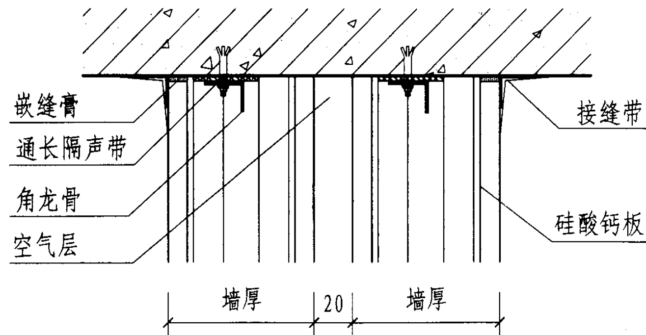
23 双层墙板与楼板顶面连接
