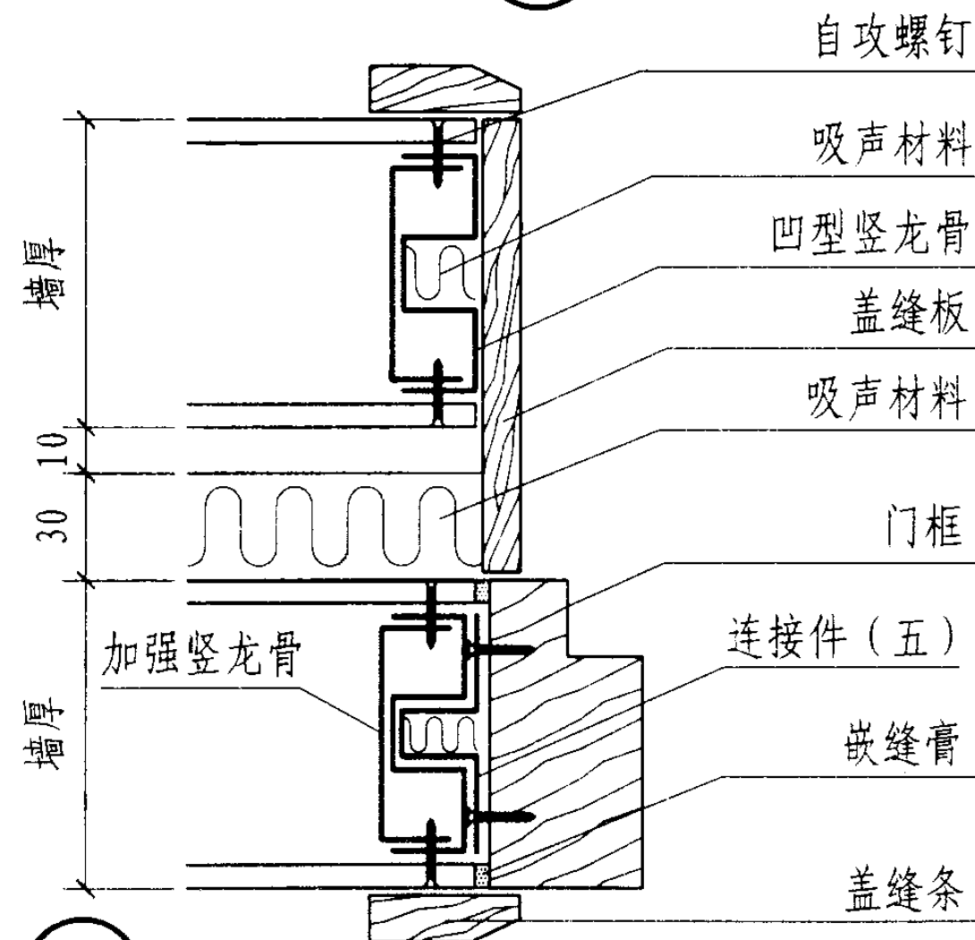
53 门框宽度 < 1000做法
